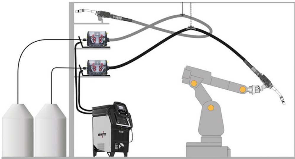
Langansyöttölaitteen- vaihtojärjestelmä
